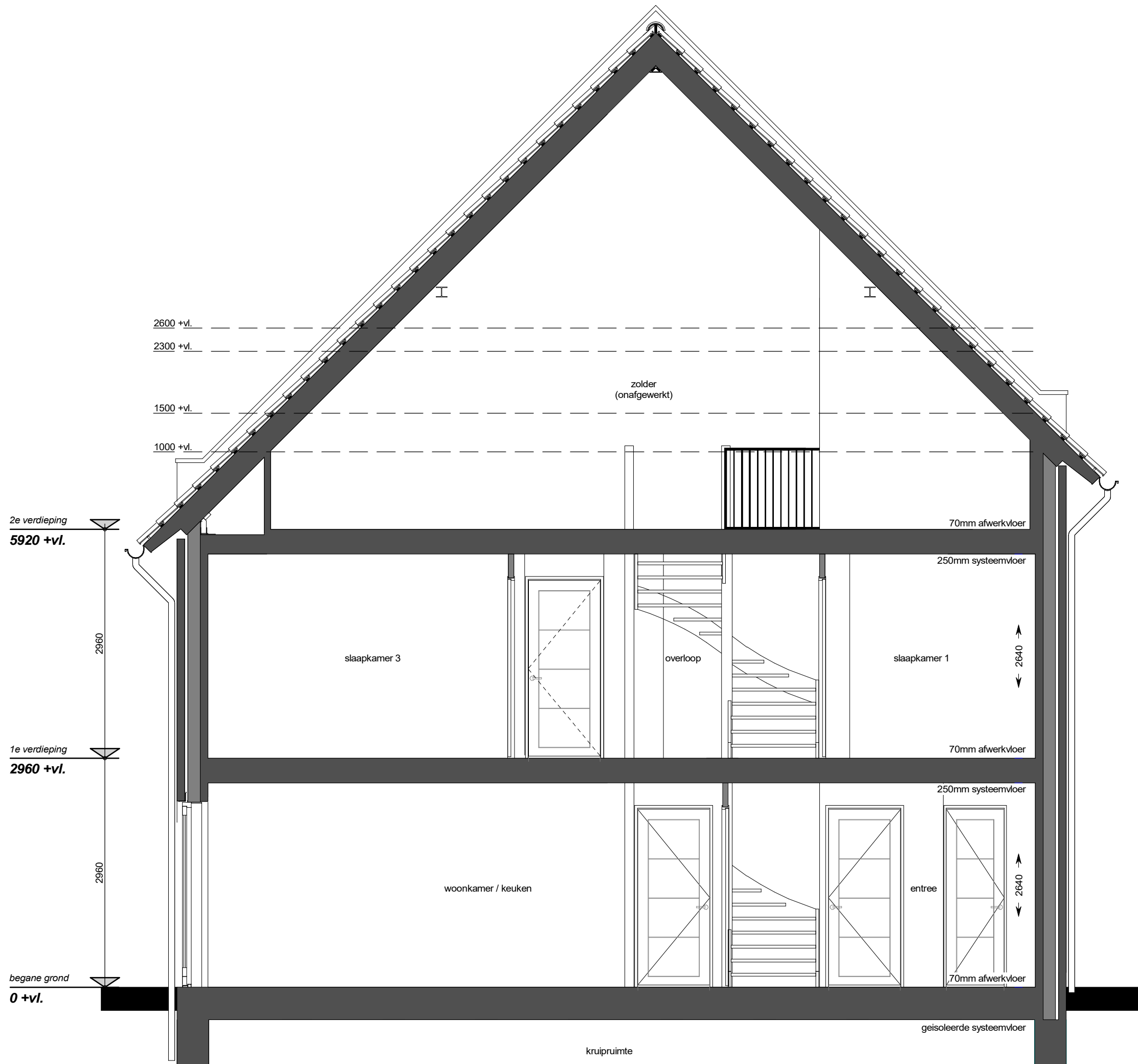
doorsnede woning
